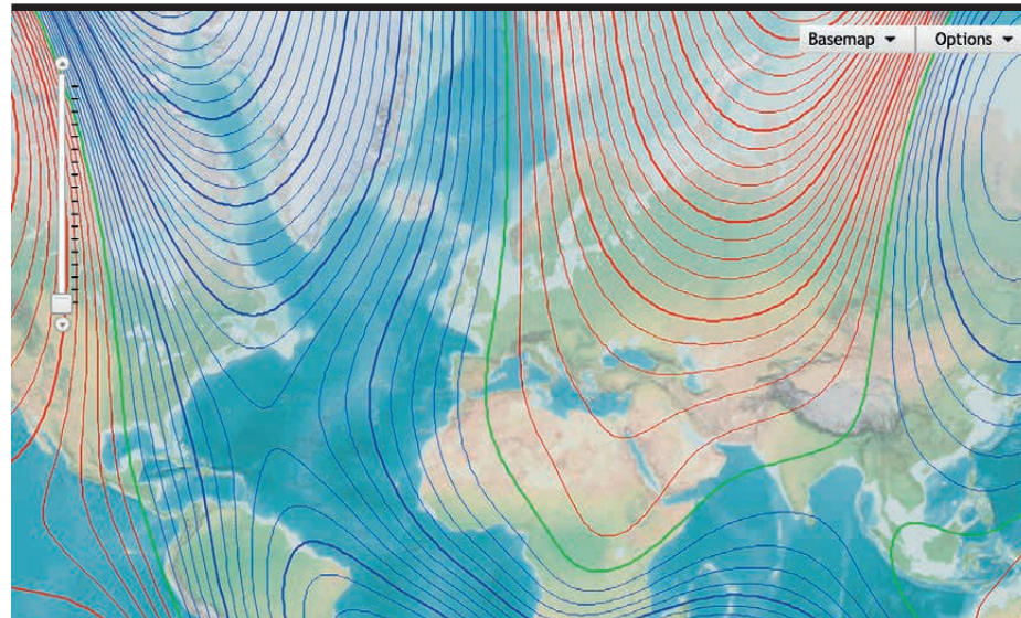
UNSICHTBARE KRAFT Das Magnetfeld der Erde. Grün eingezeichnet sind die Null-Grad-Isogene. Entlang dieser Linien existiert keinerlei Ortsmissweisung. Da die magnetischen Pole wandern, verschieben sie sich permanent, und die Missweisung verändert sich von Jahr zu Jahr
