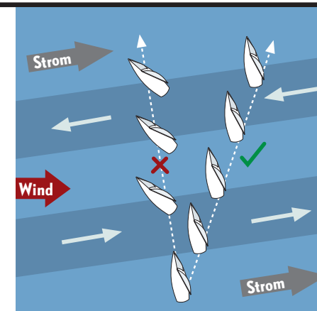
GUTE SEEMANNSCHAFT Ein Verkehrstrennungsgebiet muss in einem Winkel von 90 Grad gequert werden. Die Kollisionsverhütungsregeln beziehen sich dabei jedoch nicht auf den Kurs über Grund, sondern auf den rechtweisenden Kurs. Wer stur nach Plotter fährt, macht's also falsch
